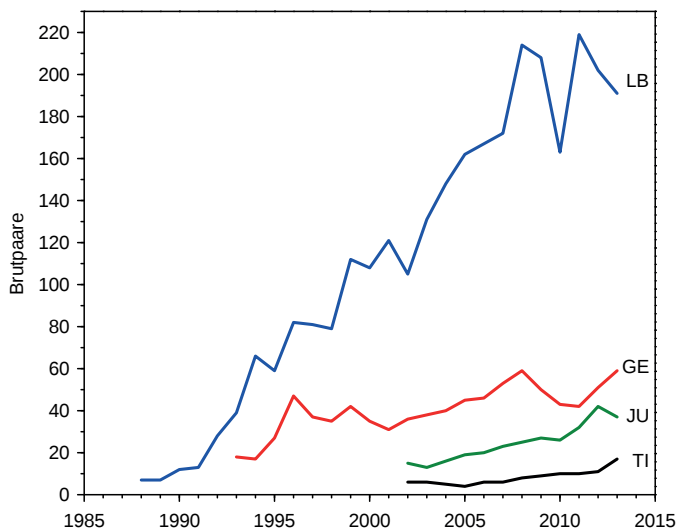
Abb. 3. Entwicklung der Bestände des Steinkäuzers in den Kantonen Genf (GE), Jura (JU) und Tessin (TI) im Vergleich mit der Entwicklung im Landkreis Ludwigsburg, Württemberg (LB). Die starke Entwicklung der Württemberger Population ist unter anderem auf die rasche räumliche Ausbreitung zurückzuführen, während sich die Schweizer Bestände nur wenig ausbreiteten. Daten freundlicherweise zur Verfügung gestellt von H. Keil, C. Meisser, A. Brahier und R. Lardelli.
